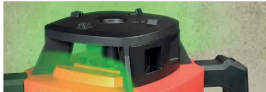
Der Anti-Reflexionsclip verhindert unerwünschte Reflexionen. (Wird bei allen Para-Modellen mitgeliefert.)
